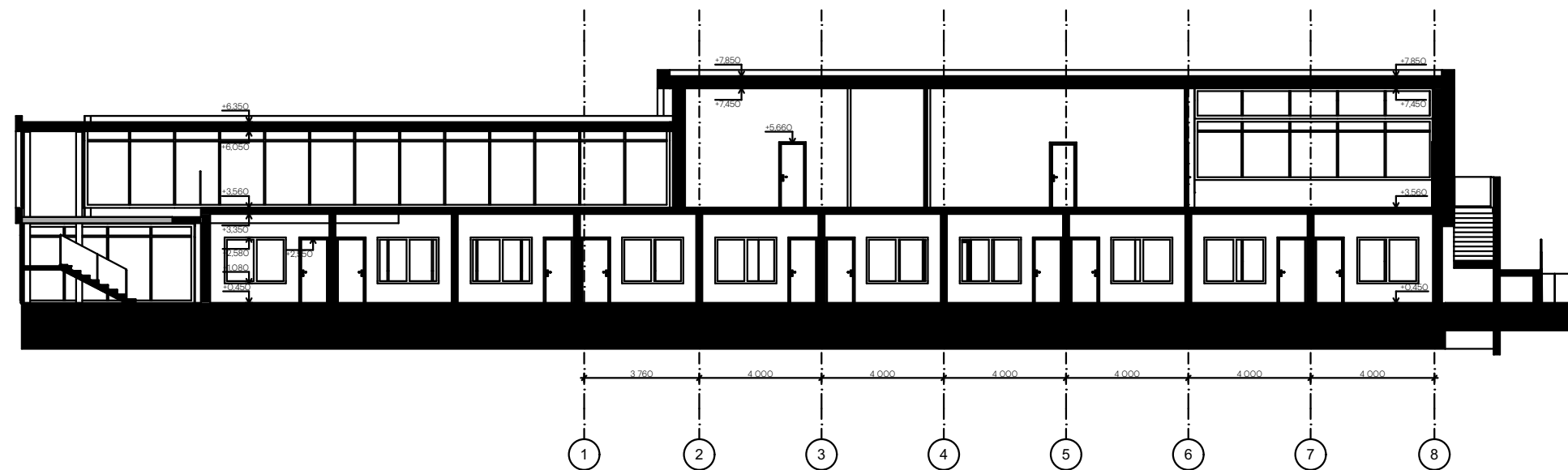
Разрез 2-2
