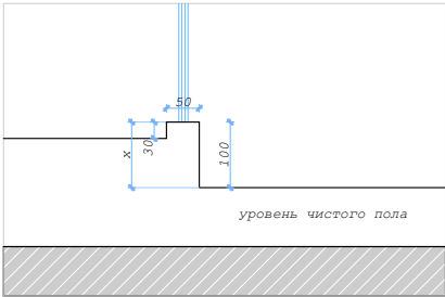
Рекомендованный узел 1. Порог душевого поддона.
