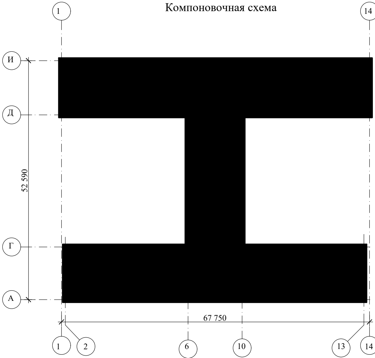
Компоновочная схема
