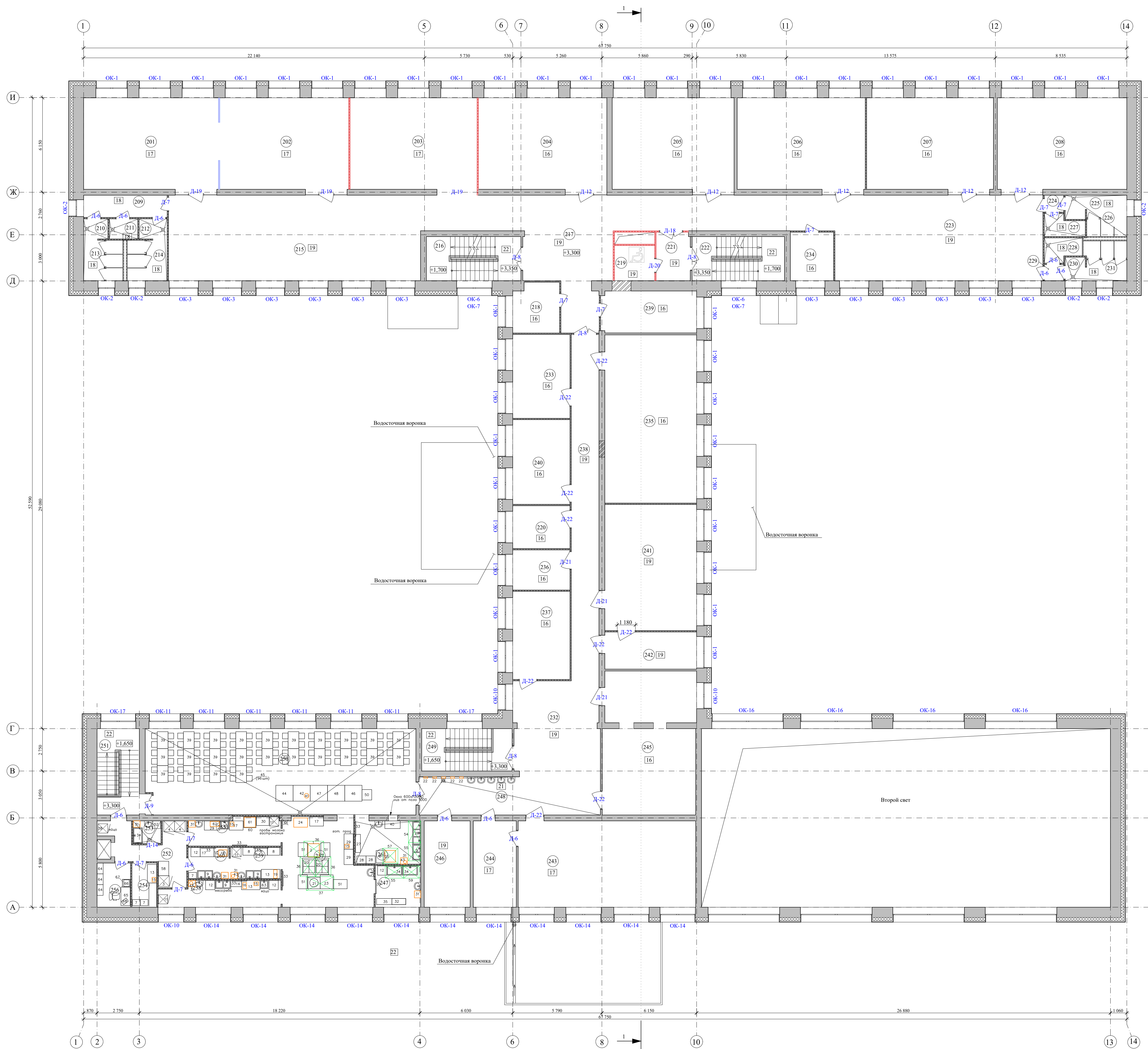
План полов и заполнения проемов 2 этажа
