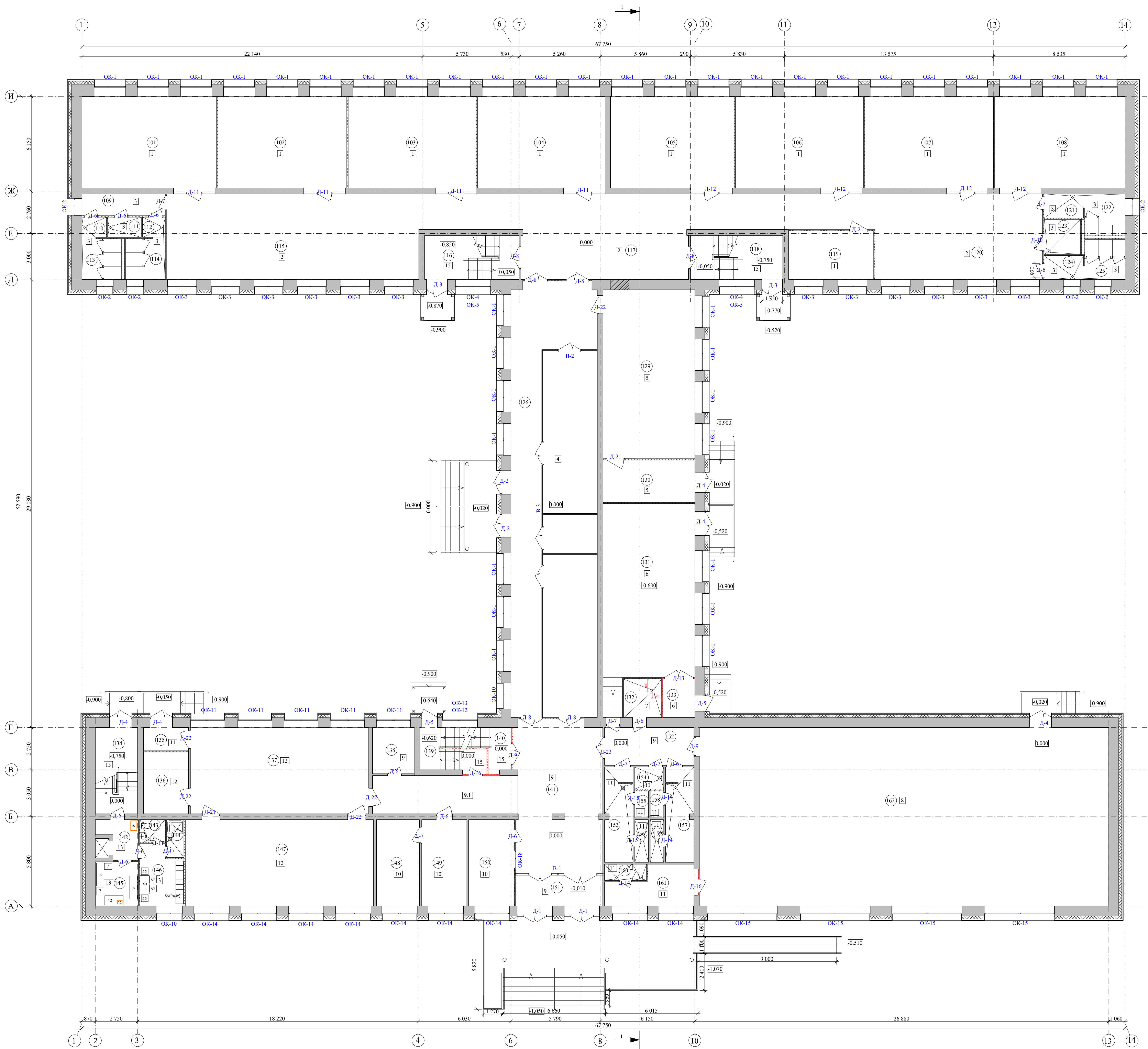
План полов и заполнения проемов 1 этажа
