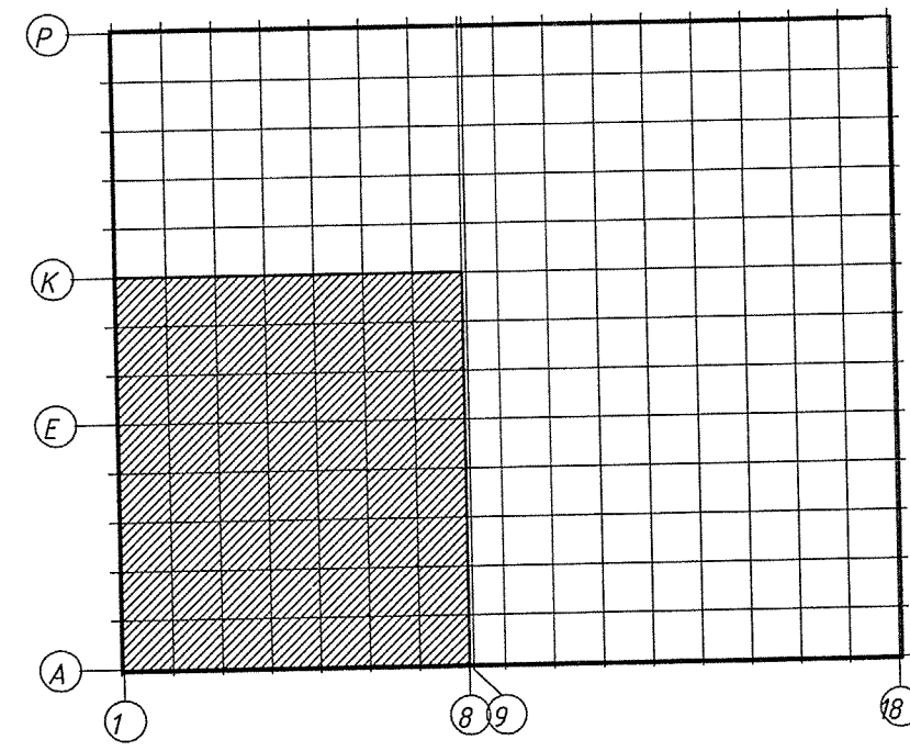
Компоновочная схема
