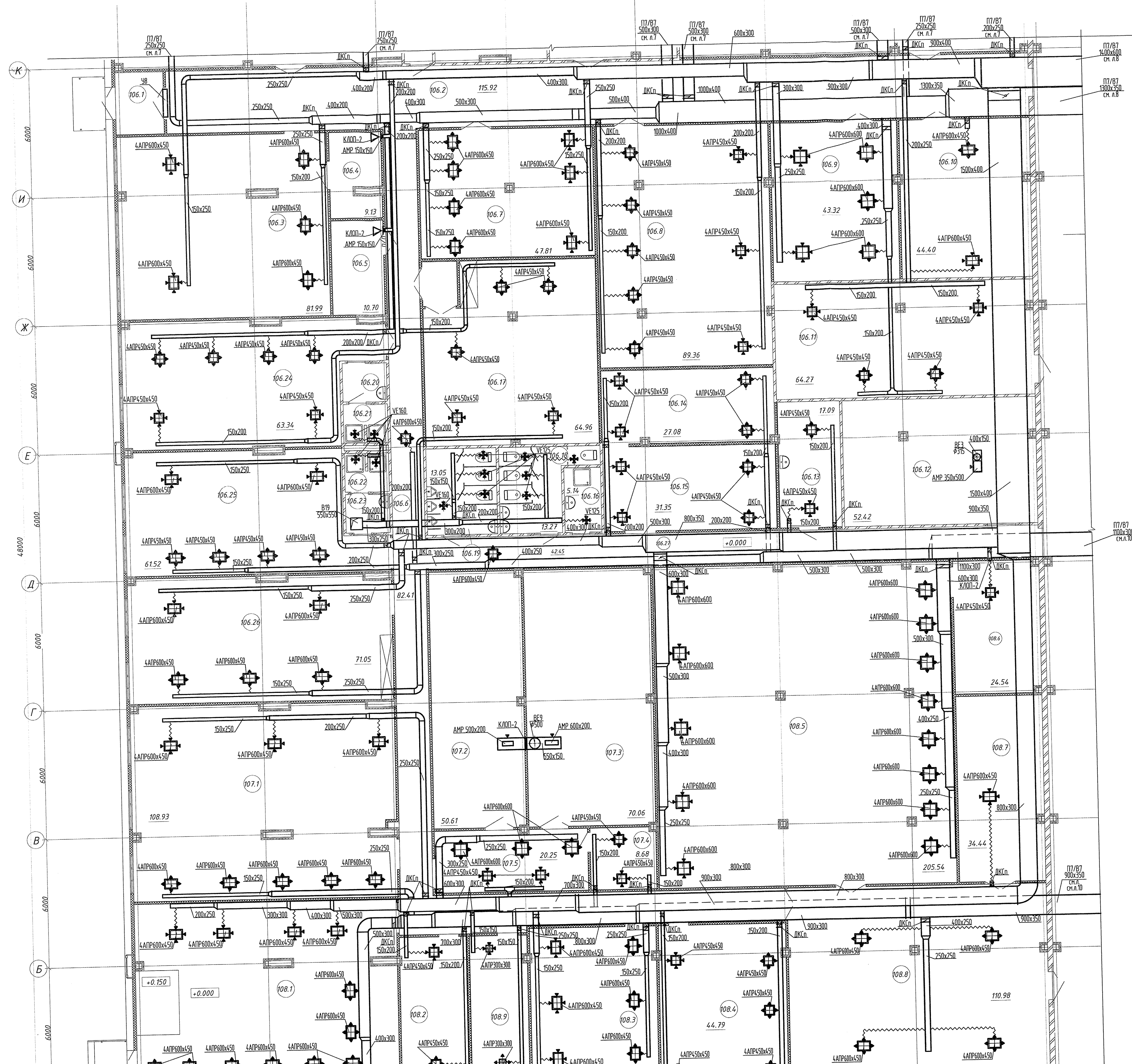
План на отм. 0.000 в осях 1-8/А-К. Вентиляция
