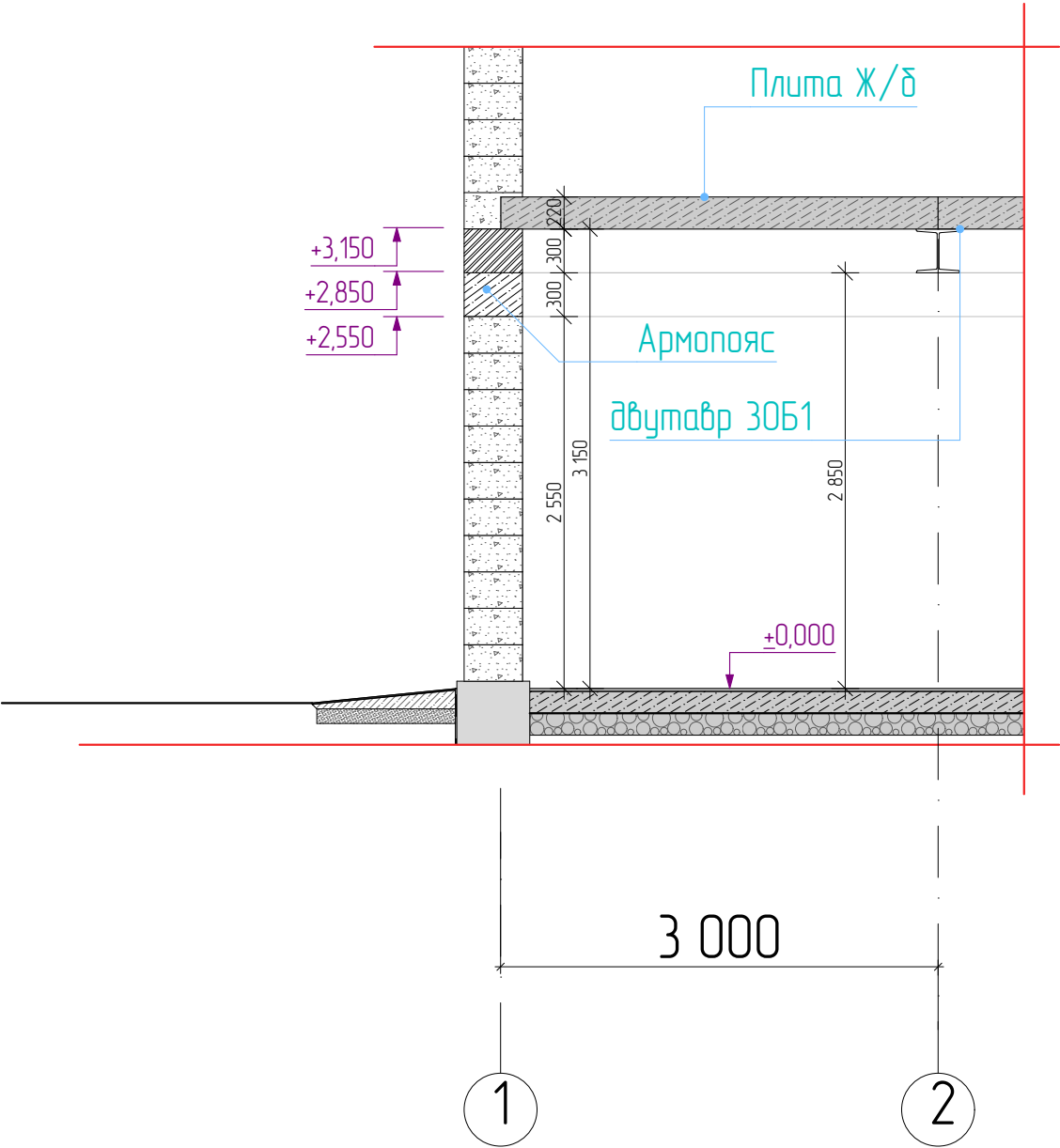
Разрез 2-2
